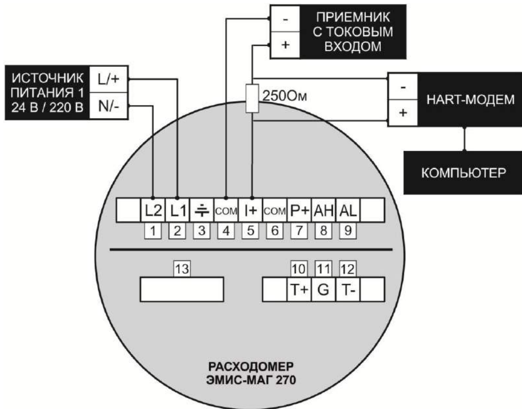
Рисунок В.5 – Схема подключения по аналоговому токовому выходному сигналу и цифровому сигналу стандарта HART
