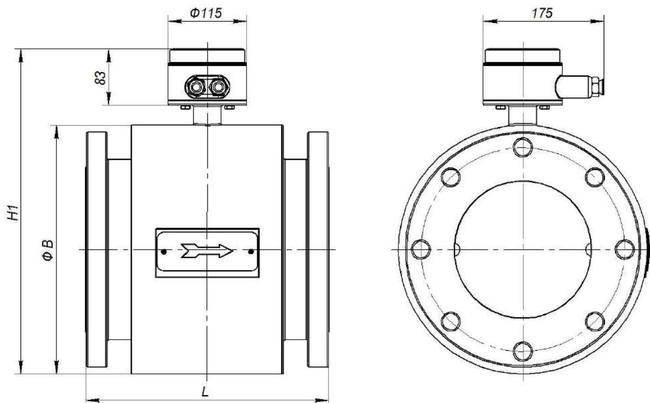
Рисунок А.3 – Габаритные и присоединительные размеры расходомера ( Dу \geq 100 мм)
