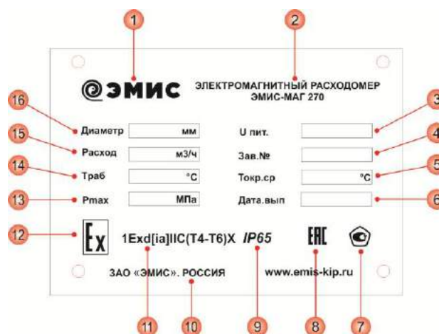
Рисунок 1.3 – Табличка расходомера
