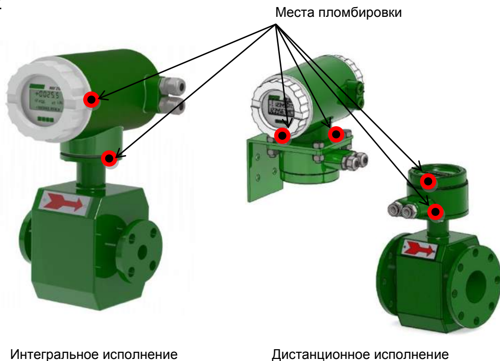
Рисунок 2.17 – Пломбирование расходомера
