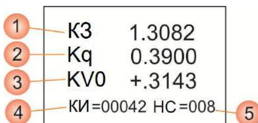
Рисунок 2.14 – Журнал изменений
