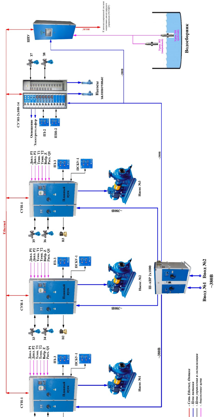
Типовая структурная схема системы управления водоотливом АСУВ «Каскад-3-Н-753-3-2-1-0-6-123-Е-УХЛ5». Для рудников, шахт и карьеров, не опасных по взрыву пыли и газа. Исполнение РН-1, степень защиты IP54.
