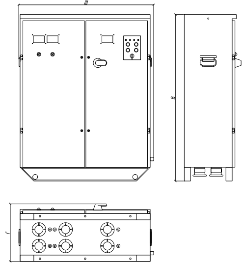
Ш-АВР-2x160-1-02М (схема №2).
