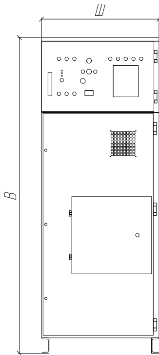
Рис. 2 Общий вид ячеек КРУ-РН.
