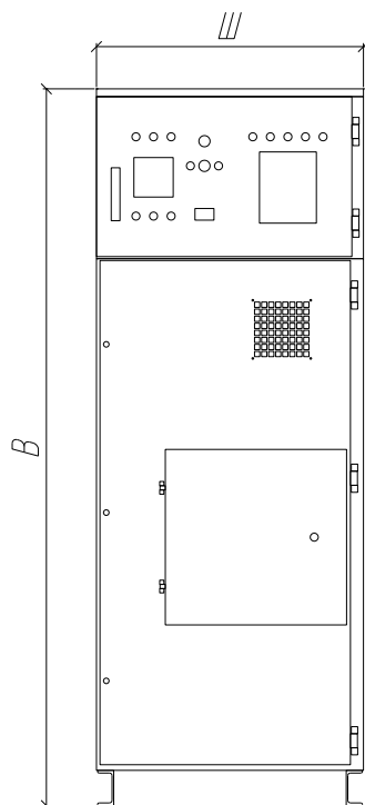
Ячейка КРУ-РН-6-ВВ-ВГ (вводная):
