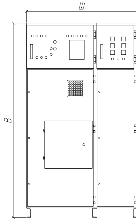
Ячейка КРУ-РН-6-ВВ-СГ (секционная):
