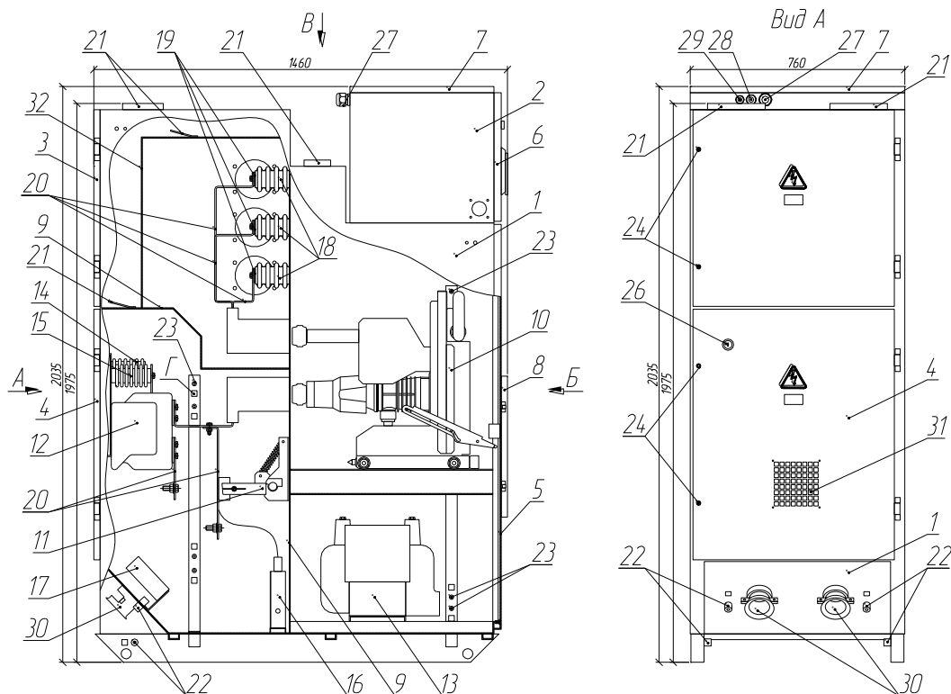
Рис. 1 Шкаф отходящих присоединений.
