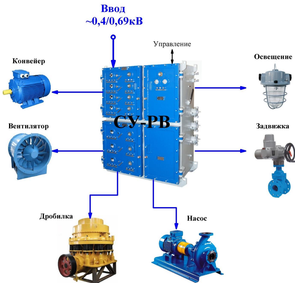
Структурная схема станции управления СУ-РВ
