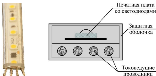
Рис.1 Конструкция светодиодной ленты ЛСР-3,6(9,6)-36.
